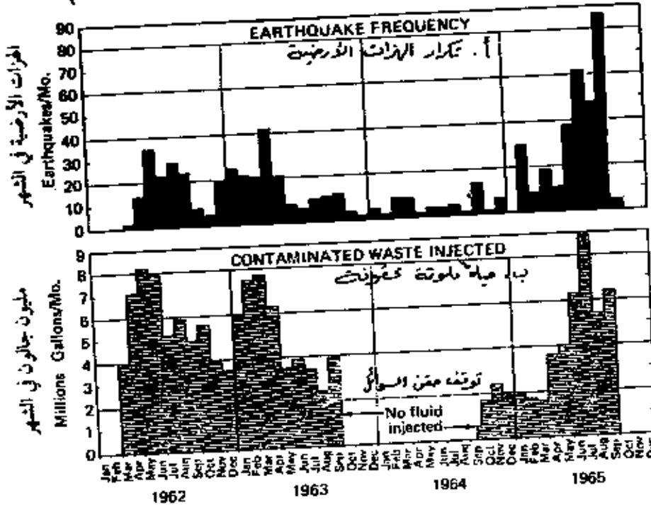
شكل (٤) : (أ) يوضح عدد الهزات الأرضية التي سجلت في الشهر في منطقة دنفر. (ب) مقدار الماء الملوث المحقون في البئر (after, Evans, 1979)
